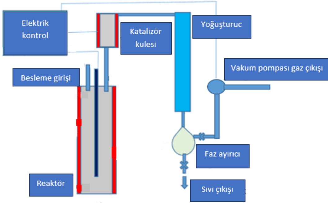
Görsel 8. Deney düzeneğinin şeması
